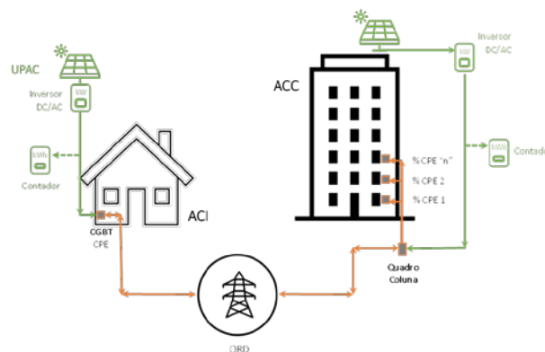
Figura 2 — Autoconsumo Individual (ACI) e Autoconsumo Coletivo (ACC)
